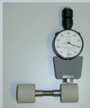
RHP 皮辊硬度测试仪
