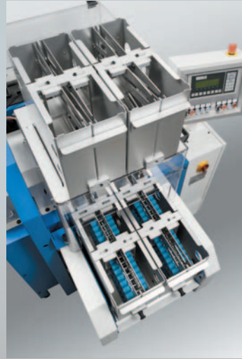
双排式皮辊储存箱
